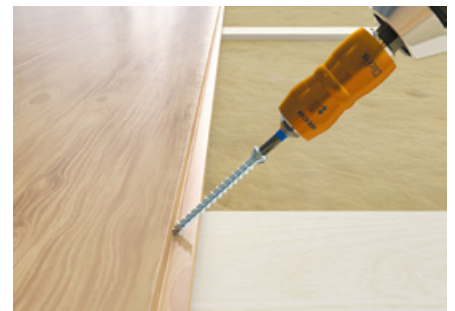
Fixierung von Dielenbelag
