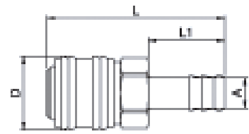
Schlauchtülle
