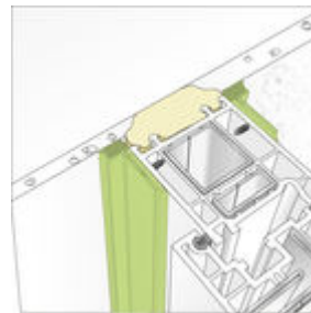
Bild 4: Ansicht der aktivierten TR450
