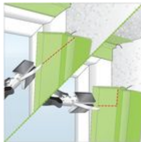
Bild1: Zuschneiden der Leiste. Abwinkeln der Leiste um 90°. Eckverbindung zuschneiden.
